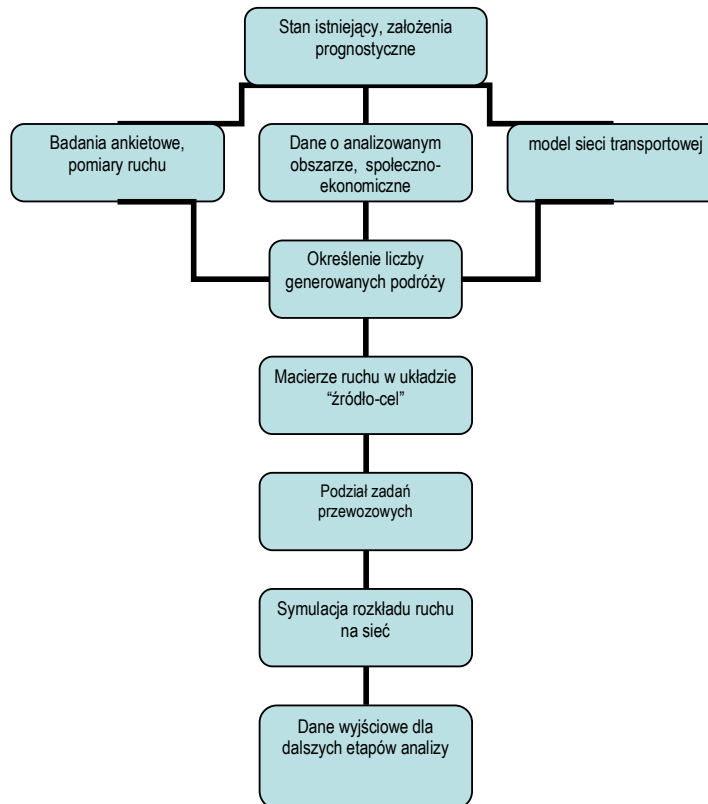
Rysunek 3 Diagram etapów prognozowania ruchu
